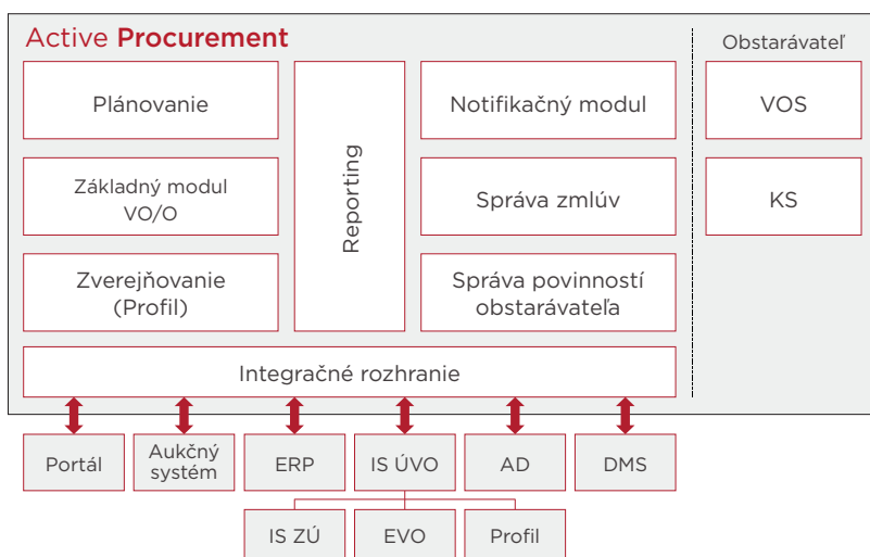
Bloková schéma informačného systému Active Procurement
